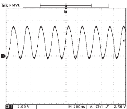
POINT (B) XL2 (Pin 14 of IC2)
