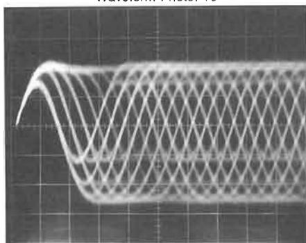
波形写真10
